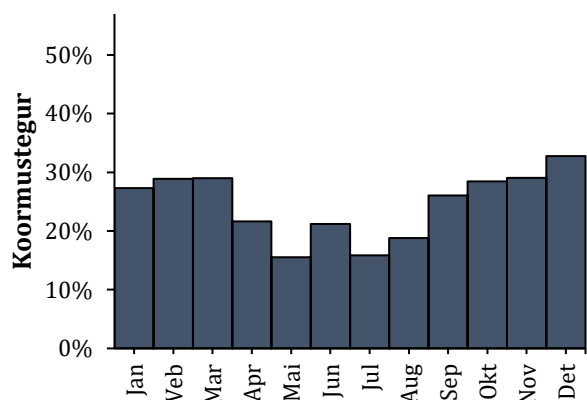
Joonis 14.17. Tuuleenergia koormustegur
