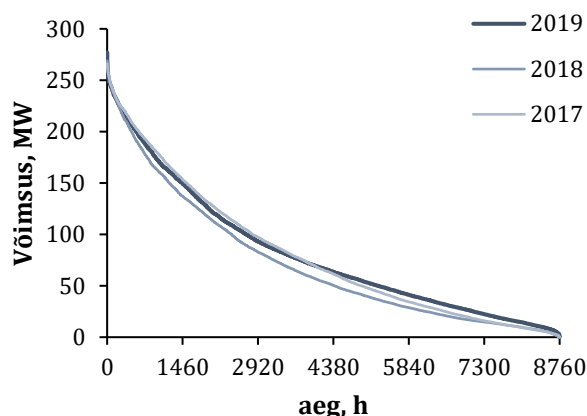
Joonis 14.16. Tuuleenergia koormusgraafik
